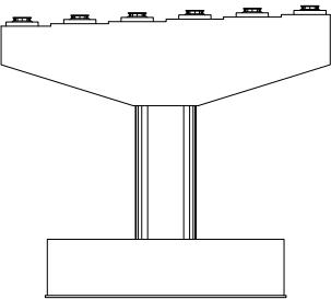
전면
