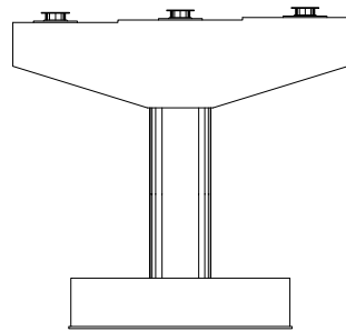
전면
