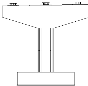
전면
